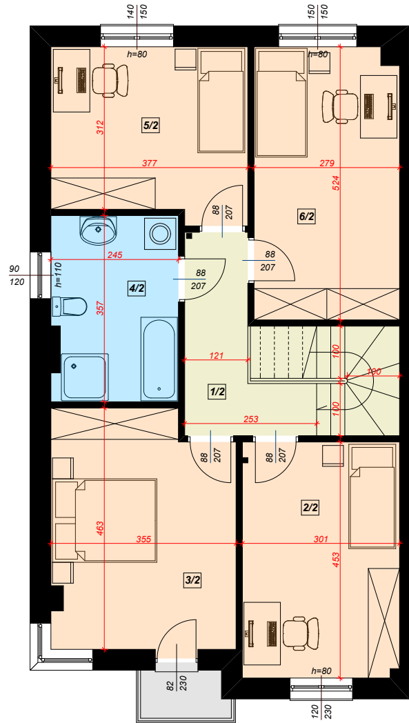
A piętro
